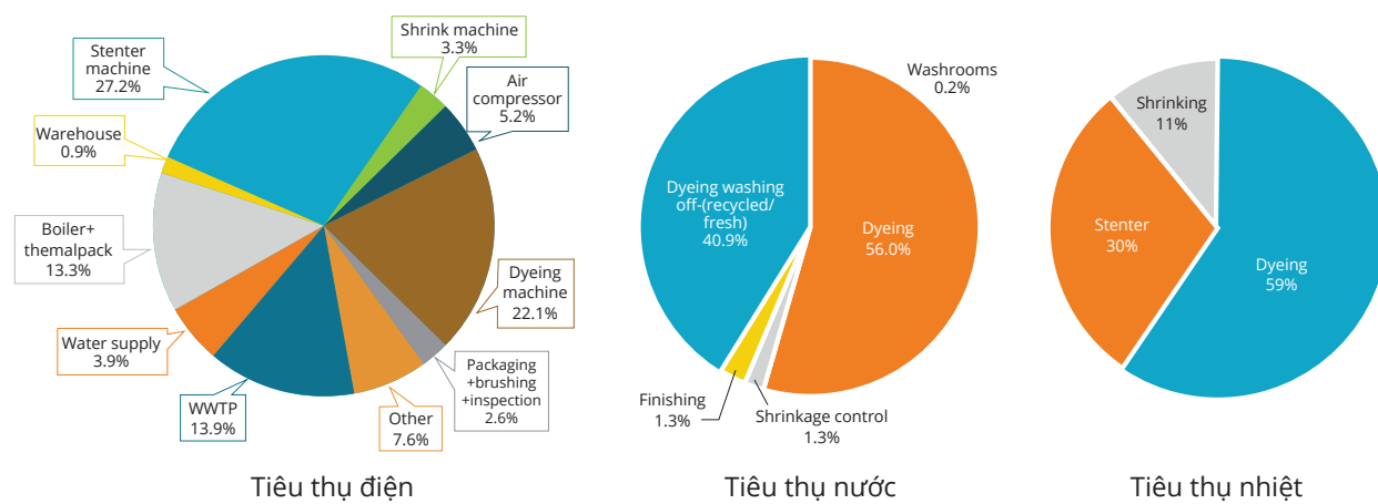
Hình 8. Cơ cấu sử dụng năng lượng trong một nhà máy dệt nhuộm điển hình
